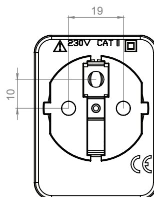
EU Socket tester
